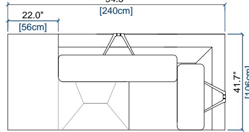
09 GRAND ANGLE/MERIDIENNE DROITE LARGE CORNER/MERIDIENNE RIGHT GRAN ANGULO/MERIDIENNE DERECHA 94.5"
