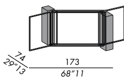
basamento - base S2W
