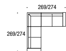
Art. BR+09+09+AQ+09+09+BR N. 4 poltrone + n. 2 braccioli + angolo quadro N. 4 armchairs + n. 2 armrests + square corner N. 4 chaufeuse + N. 2 accoudoirs + angle carré
