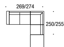
Art. BR+09+09+AQ+13+09 N. 3 poltrone + bracciolo + angolo quadro + pouff N. 3 armchairs + armrest + square corner + pouf N. 3 chaufeuses + accoudoir + angle carré + pouf
