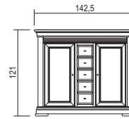
VOL. 0,999 m 3 GR.W. 115 Kg. Prof. - Depth 50 cm. Comò uomo 2 ante + 5 cassetti Gentleman's chest w/2 drs + 5 drws Cd. 326861/10 € 2.038,00
