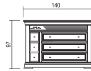
VOL. 0,873 m 3 GR.W. 109 Kg. Prof. - Depth 55 cm. Comò 7 cassetti Dresser, 7 drawers Cd. 326831/10 € 1.836,00
