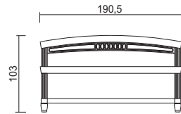
VOL. 0,272 m 3 GR.W. 62,5 Kg. Prof. - Depth 207 cm. Letto (dim. int. 180 x 200) Bed (int. dim. 180 x 200) Cd. 327852 € 1.541,00
