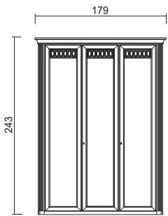
VOL. 0,963 m 3 GR.W. 202 Kg. Prof. - Depth 68,5 cm. Armadio 3AP Wardrobe, 3 doors Cd. 327803/5 € 2.623,00
