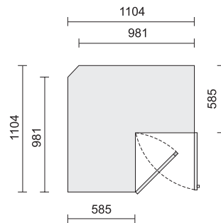
Pianta - Plan
