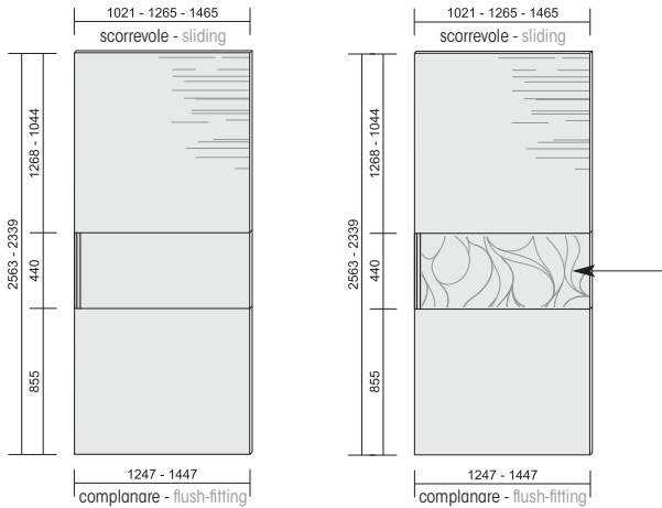
sezione - section
