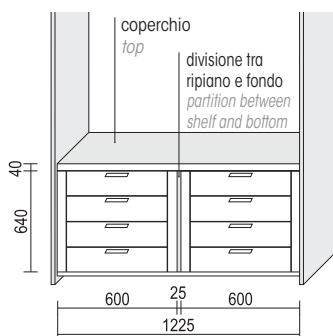
ES. DI DUE CASSETTIERE AFFIANCATE EX. OF TWO PAIRED INTERNAL DRAWER UNITS
