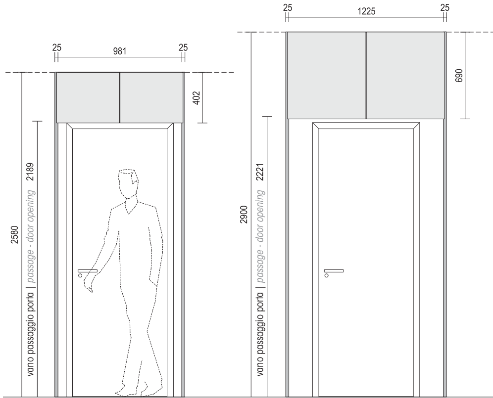
Esempi di ponte sopra un passaggio o una porta | Examples of span unit over a passage or a door
