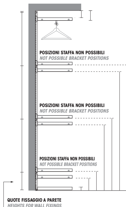
DIMENSIONE MINIMA DI POSIZIONAMENTO MINIMUM SPACE REQUIREMENTS
