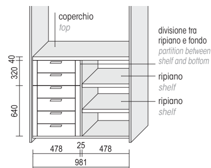
ES. DI CASSETTIERA + RIPIANI LATERALI EX. OF INTERNAL DRAWER UNIT + SIDE SHELVES
