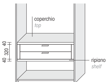
ES. DI CASSETTIERA SOPRA RIPIANO (massimo 2 cassetti) EX. OF INTERNAL DRAWER UNIT ON SHELF (max 2 drawers)
