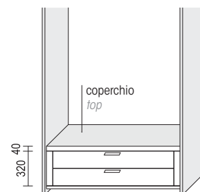
ES. DI CASSETTIERA APPOGGIATA AL FONDO EX. OF INT. DRAWER UNIT RESTING ON BOTTOM
