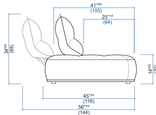
CHAUFFEUSE - DOSSIER AVEC MECANISME A BALANCIER GRAND DEBATTEMENT ARMLESS CHAIR - BACKREST WITH LONG PATH MECHANISM CHAUFFEUSE - RESPALDO CON MECANISMO MOVIMIENTO AMPLIO
