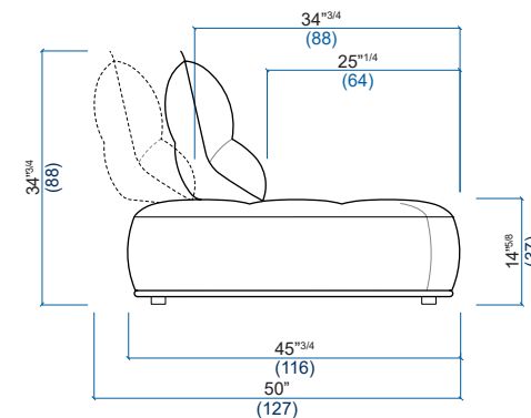
CHAUFFEUSE - DOSSIER AVEC MECANISME A BALANCIER PETIT DEBATTEMENT ARMLESS CHAIR - BACKREST WITH SHORT PATH MECHANISM CHAUFFEUSE - RESPALDO CON MECANISMO MOVIMIENTO CORTO
