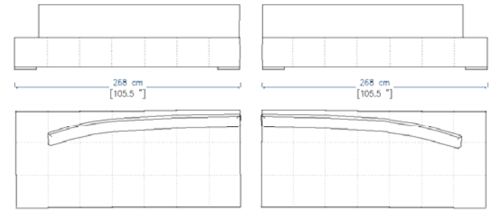
GRAND TERMINAL GAUCHE LARGE END UNIT LEFT GRAN TERMINAL IZQUIERDO
