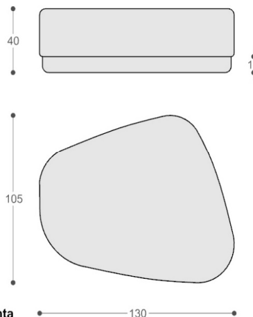
Pianta Plan
