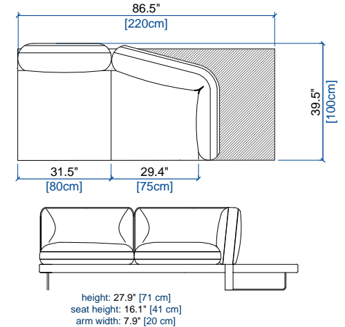
176 BANQUETTE 3 PLACES - TROTTOIR DROIT 3-SEAT ARMLESS SOFA - RIGHT PLATFORM ELEMENTO 3 PLAZAS - PLATAFORMA DERECHA
