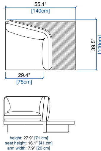
180 BANQUETTE 1,5 PLACE - TROTTOIR DROIT 1.5-SEAT ARMLESS SOFA - RIGHT PLATFORM BANQUETA 1,5 PLAZA - PLATAFORMA DERECHA
