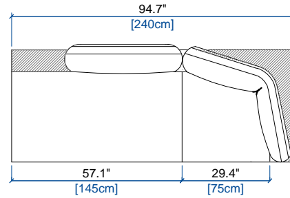
09 GRAND ANGLE/MERIDIENNE DROITE LARGE CORNER/MERIDIENNE RIGHT GRAN ANGULO/MERIDIENNE DERECHA
