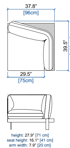
28 BATARD 1 PL. ACC. DROIT 1-SEAT 1-ARM UNIT RIGHT ARMREST BATARD 1 PL. APOY. DERECHO
