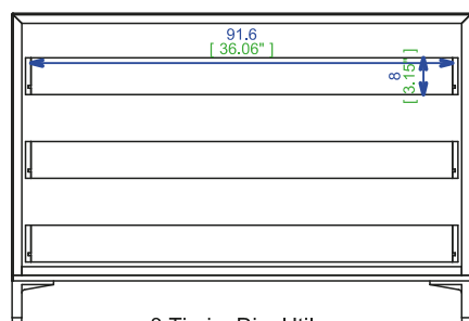
3 Tiroirs Dim Utiles 916 x 376 x 80 mm
