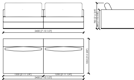
ELEMENTO SENZA BRACCIOIU / ELEMENT WITHOUT ARMS_240X105 2 SEDUTE DA 120 / 2 SEATS 120
