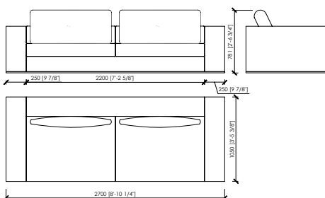
DIVANO 2 POSTI / 2 SEATER SOFA_270X105 2 SEDUTE DA 100 / 2 SEATS 110
