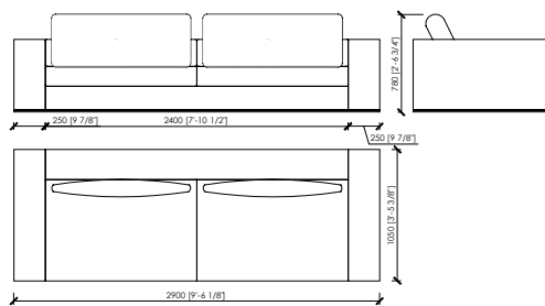
DIVANO 2 POSTI / 2 SEATER SOFA_290X105 2 SEDUTE DA 100 / 2 SEATS 110
