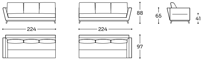
PFD - 153 / PFD - 154
