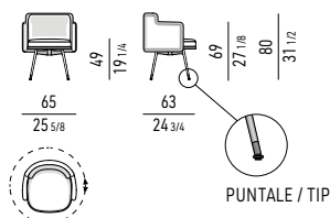
MOVIMENTO GIREVOLE 360° CON RITORNO 360° SWIVEL MOVEMENT WITH RETURN
