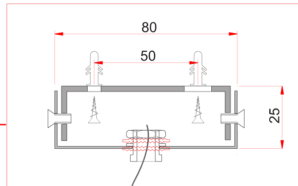
Anello Interno/Inner Ring
